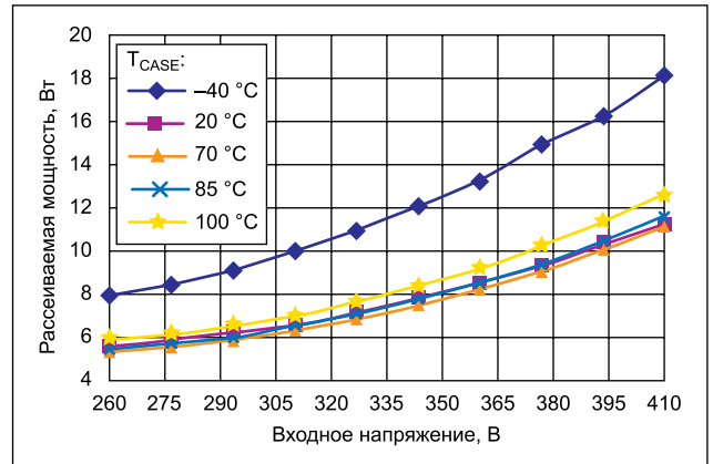
Рис. 3. Графики зависимости мощности, рассеиваемой модулем VI BCM в режиме холостого хода, от входного напряжения модуля и температуры корпуса T CASE
