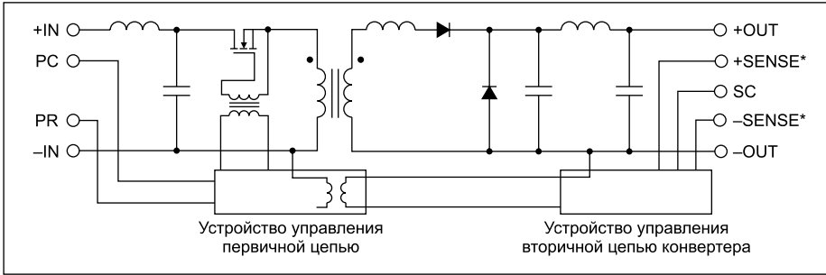
Рис. 2. Упрощенная функциональная схема конвертеров семейств MaxI и Mini
