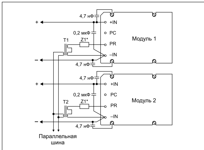
Рис. 6. Синхронизация модулей в режиме Power Sharing через интерфейс с трансформаторной связью
