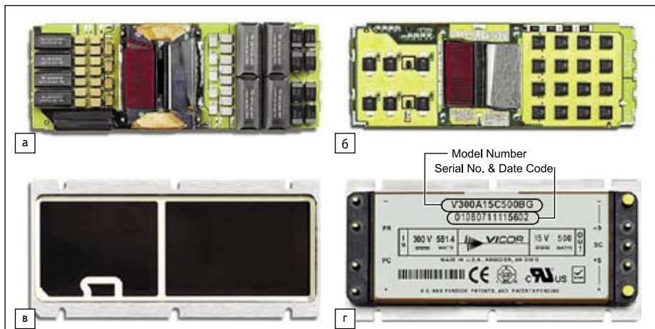
Рис. 3. Конструкция модуля второго поколения: а) плата (вид сверху); б) плата (вид снизу); в) основание модуля (внутренняя сторона); г) модуль в сборе
