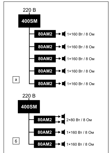
Рис. 8. Примеры приложений на основе серии ICEmatch: а) домашний кинотеатр; б) 4-полосная активная акустическая система
