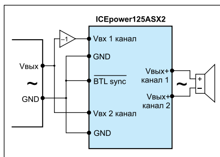
Рис. 2. Включение усилителя в мостовом режиме (BTL)
