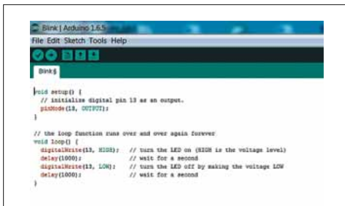
Рис. 4. Стандартный пример управления светодиодом
