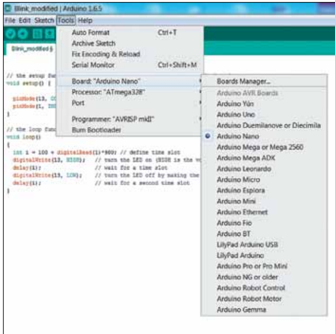
Рис. 3. Установка типа платы в Arduino IDE
