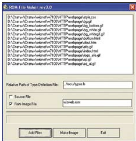
Рис. 5. Утилита ROMFILEMaker.exe
